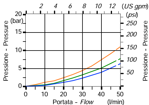
Perdite di carico P⇒T P⇒T pressure drop
