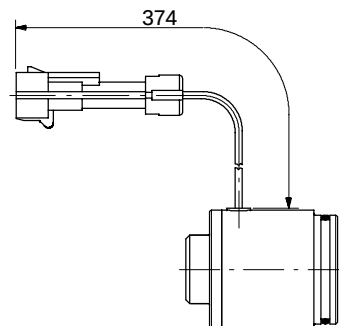
Bobina con connessione Packard M-Pack
