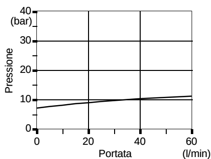
Curva caratteristica
