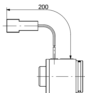
Bobina con connessione AMP Fastin-Faston
