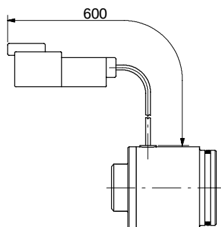
Bobina con connessione Deutsch DT
